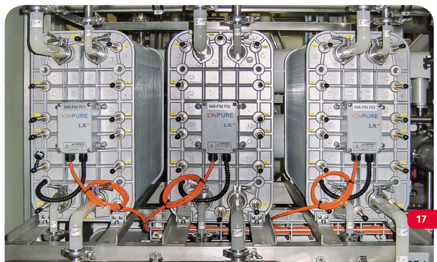
Hohe Reinstwasserqualität mit Elektrodeionisation
